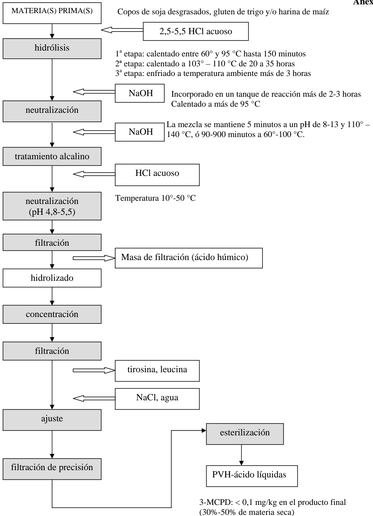
Fig: Proceso de fabricación de PVH-ácido a escala comercial
